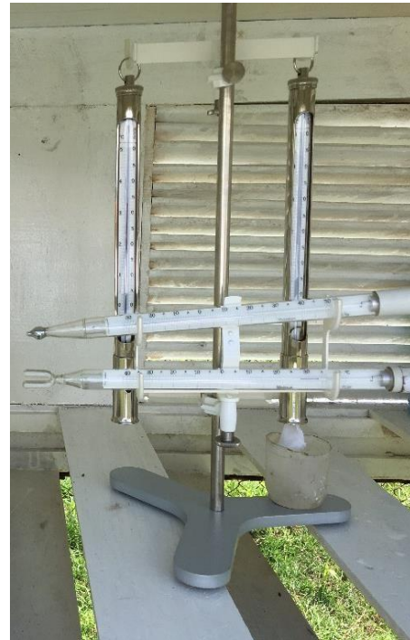
Termómetros Extremos y Comunes
