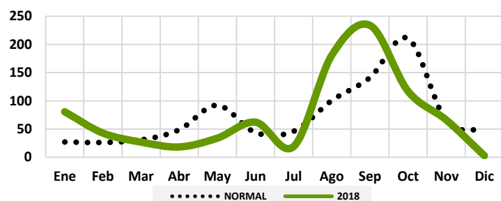
Gráfico 38: Comportamiento precipitaciones La Romana
