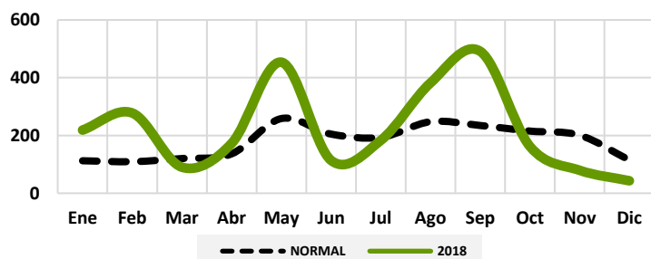
Gráfico 48: Comportamiento precipitaciones Villa Altagracia
