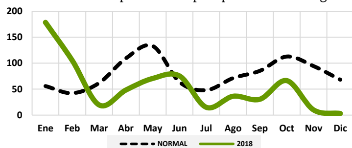
Gráfico 90: Comportamiento precipitaciones Santiago/Licey
