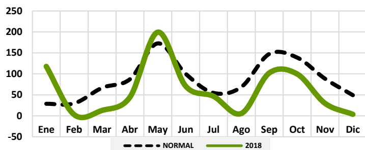
Gráfico 66: Comportamiento precipitaciones Barahona
