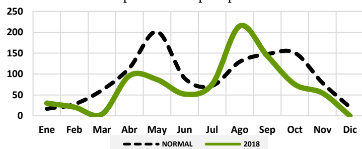
Gráfico 64: Comportamiento precipitaciones El Cercado.
