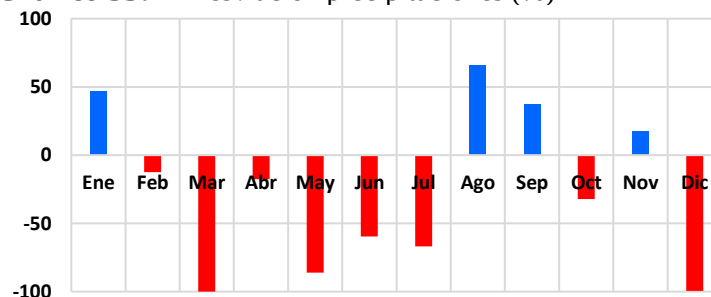
Gráfico 53: Desviación precipitaciones (%)
