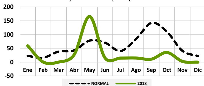
Gráfico 58: Comportamiento precipitaciones Azua
