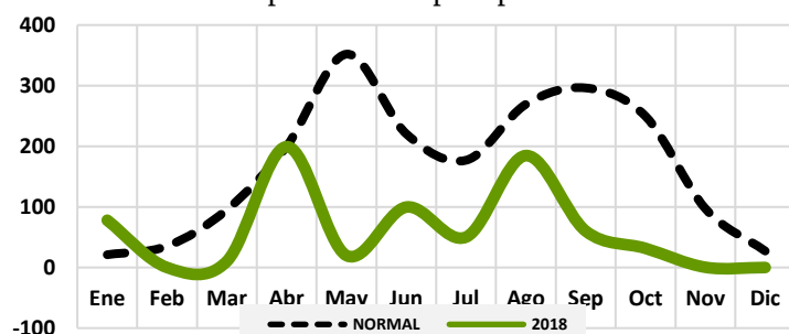
Gráfico 60: Comportamiento precipitaciones Elías Piña.
