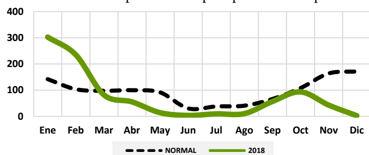
Gráfico 96: Comportamiento precipitaciones Luperón/Puerto Plata
