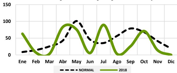
Gráfico 68: Comportamiento precipitaciones Neyba.
