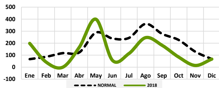
Gráfico 50: Comportamiento precipitaciones Monte Plata
