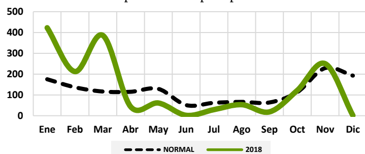
Gráfico 94: Comportamiento precipitaciones La Unión/Puerto Plata
