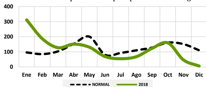
Gráfico 74: Comportamiento precipitaciones La Vega
