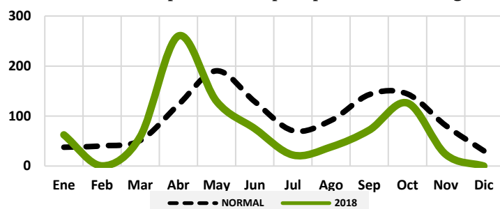
Gráfico 102: Comportamiento precipitaciones Santiago Rodríguez
