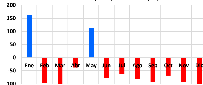
Gráfico 59: Desviación precipitaciones (%)
