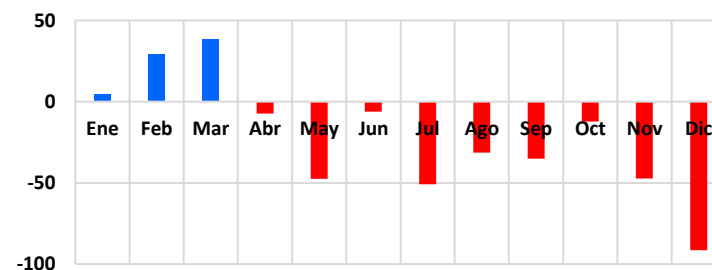
Gráfico 35: Desviación precipitaciones (%)
