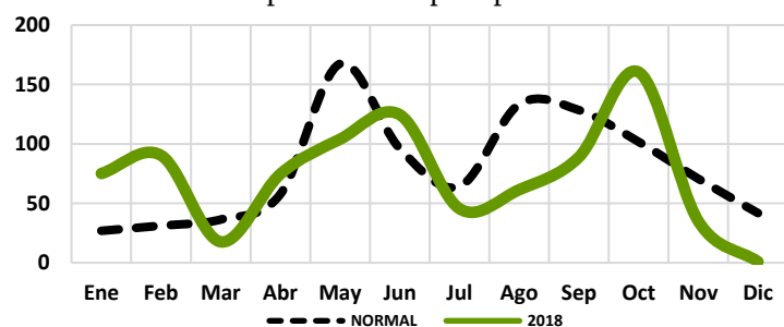
Gráfico 80: Comportamiento precipitaciones Constanza.
