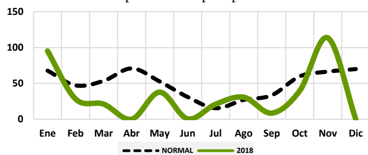
Gráfico 106: Comportamiento precipitaciones Montecristi
