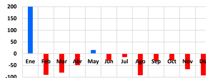
Gráfico 67: Desviación precipitaciones (%)
