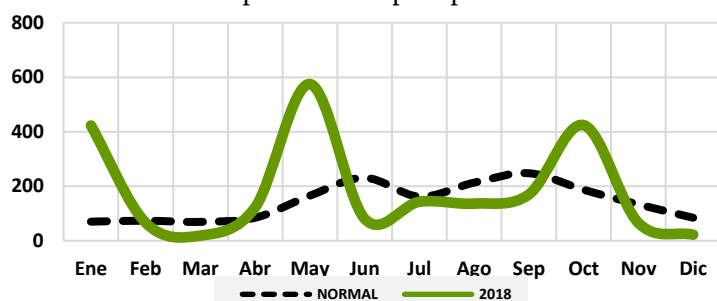
Gráfico 72: Comportamiento precipitaciones Polo.
