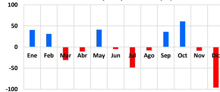
Gráfico 89: Desviación precipitaciones (%)
