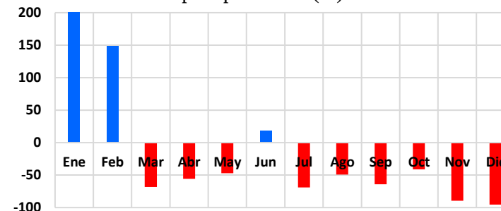
Gráfico 91: Desviación precipitaciones (%)
