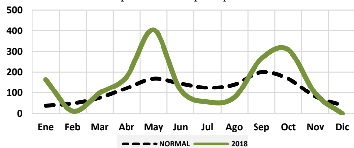
Gráfico 108: Comportamiento precipitaciones Loma de Cabrera
