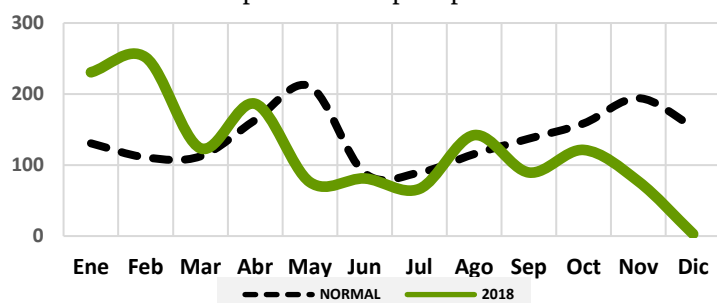
Gráfico 82: Comportamiento precipitaciones Jarabacoa
