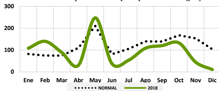
Gráfico 36: Comportamiento precipitaciones Higüey
