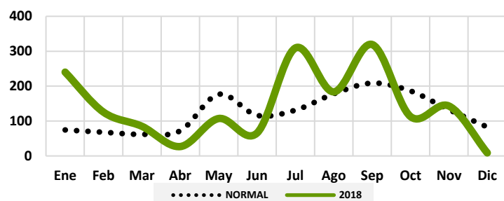
Gráfico 42: Comportamiento precipitaciones Santo Domingo
