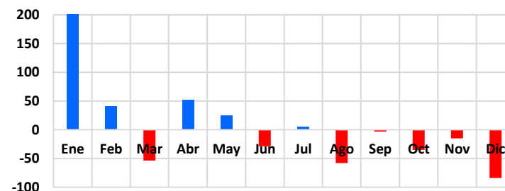
Gráfico 45: Desviación precipitaciones (%)
