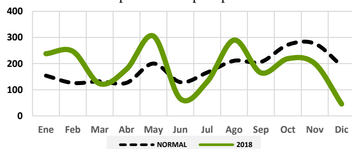
Gráfico 84: Comportamiento precipitaciones Samaná.
