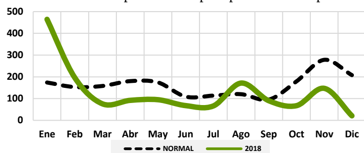
Gráfico 98: Comportamiento precipitaciones Gaspar Hernández
