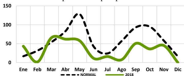
Gráfico 70: Comportamiento precipitaciones Jimaní
