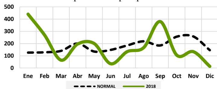
Gráfico 78: Comportamiento precipitaciones Juma/Bonao
