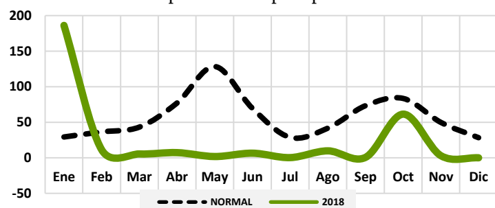
Gráfico 100: Comportamiento precipitaciones Mao
