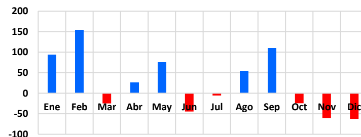
Gráfico 49: Desviación precipitaciones (%)
