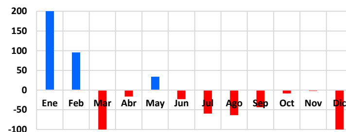
Gráfico 47: Desviación precipitaciones (%)
