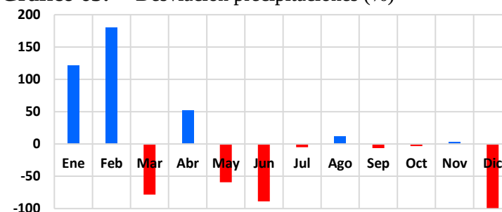
Gráfico 63: Desviación precipitaciones (%)
