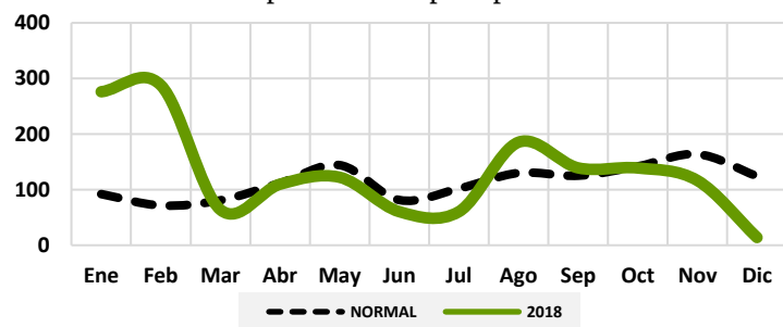
Gráfico 76: Comportamiento precipitaciones Salcedo.
