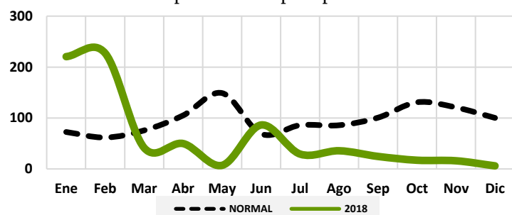
Gráfico 92: Comportamiento precipitaciones Moca.
