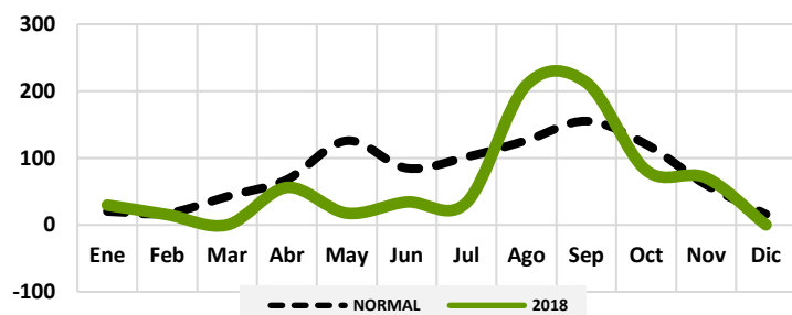
Gráfico 56: Comportamiento precipitaciones San Juan De La Mag.
