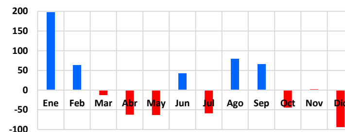
Gráfico 39: Desviación precipitaciones (%)
