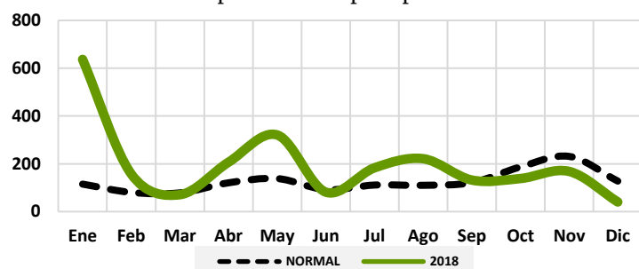
Gráfico 86: Comportamiento precipitaciones Cabrera
