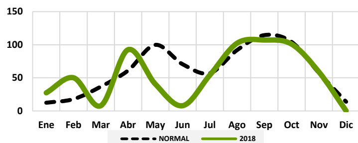
Gráfico 62: Comportamiento precipitaciones Padre Las Casas
