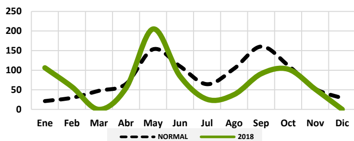
Gráfico 46: Comportamiento precipitaciones San José de Ocoa
