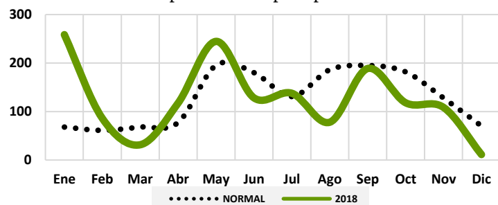
Gráfico 44: Comportamiento precipitaciones San Cristóbal
