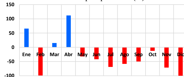
Gráfico 103: Desviación precipitaciones (%)
