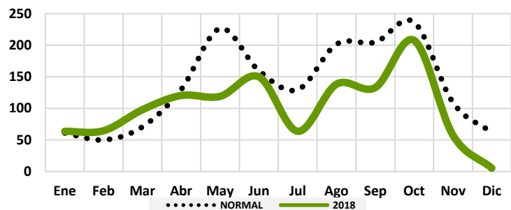
Gráfico 34: Comportamiento precipitaciones Hato Mayor
