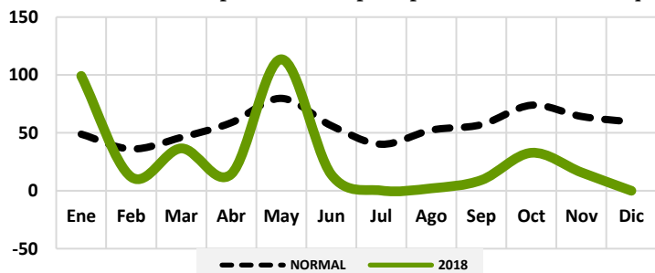
Gráfico 104: Comportamiento precipitaciones Villa Vásquez
