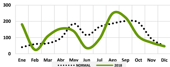
Gráfico 40: Comportamiento precipitaciones San José de los Llanos
