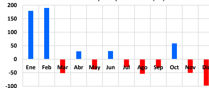
Gráfico 81: Desviación precipitaciones (%)
